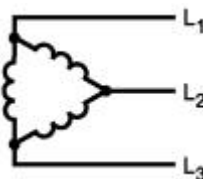
Соединение треугольником
