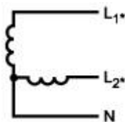
Фазовый угол - 90°
