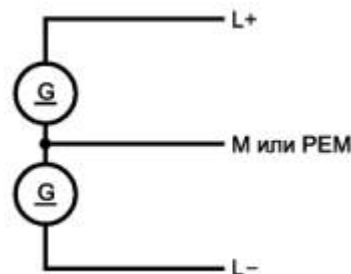
Рисунок 7 - Трехпроводная система
